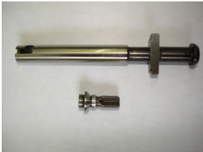
Élément de pompage et clapet de refoulement
